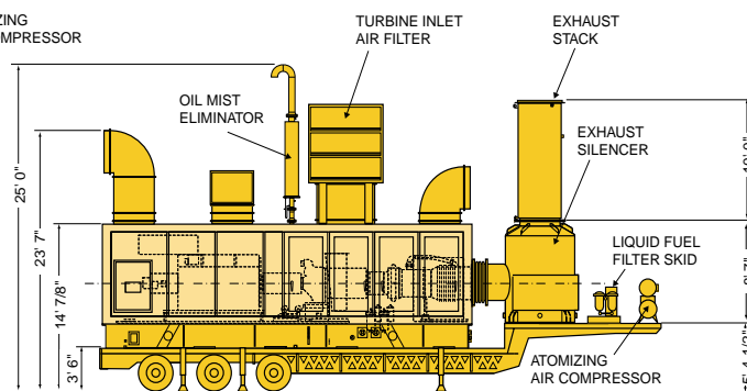
GENERATOR MODULE
